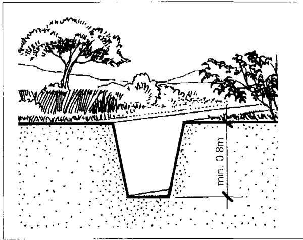
field/bush min. 0.8 m
