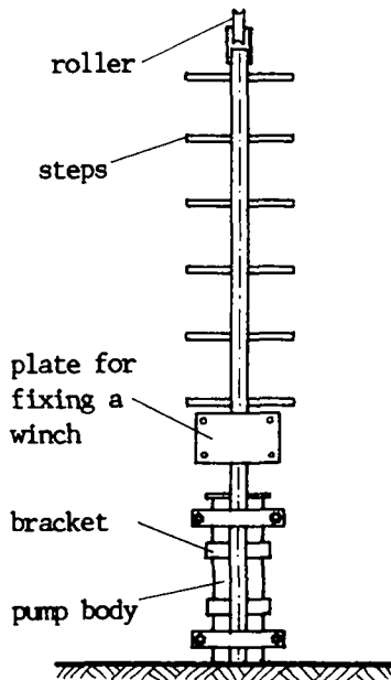
SIDE-VIEW A-A
