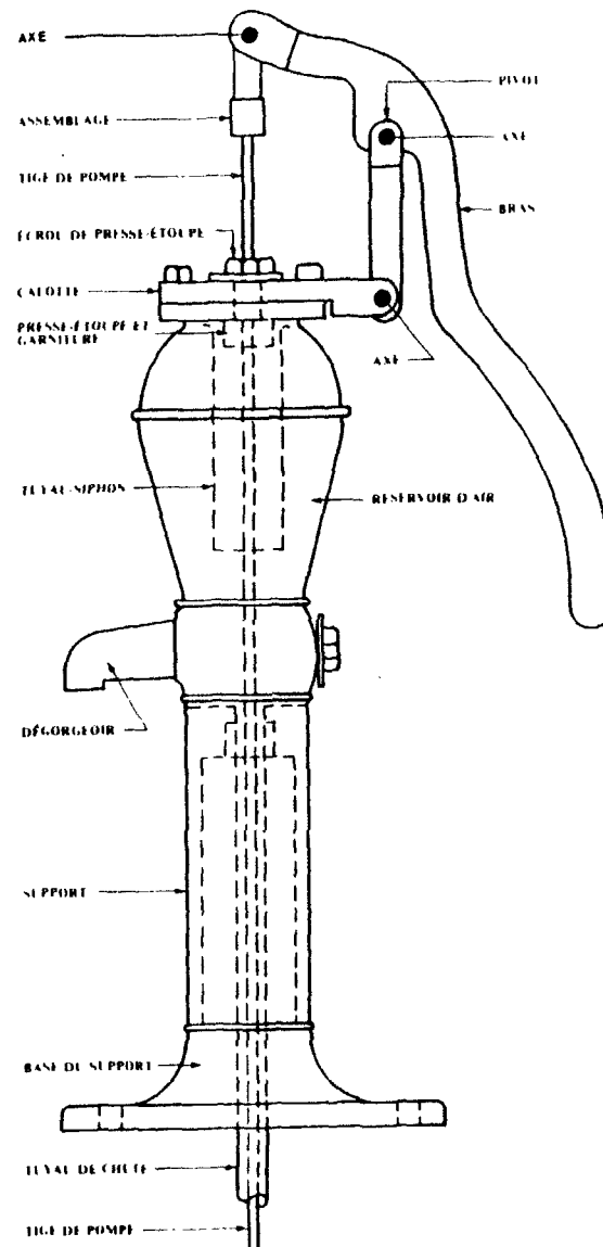
POMPE A MAIN MUNIE D'UN PRESSE-ETOUPE ET D'UNE TIGE DE POMPE GUIDEE POUVANT ETRE UTILISEE COMME POMPE FOULANTE
