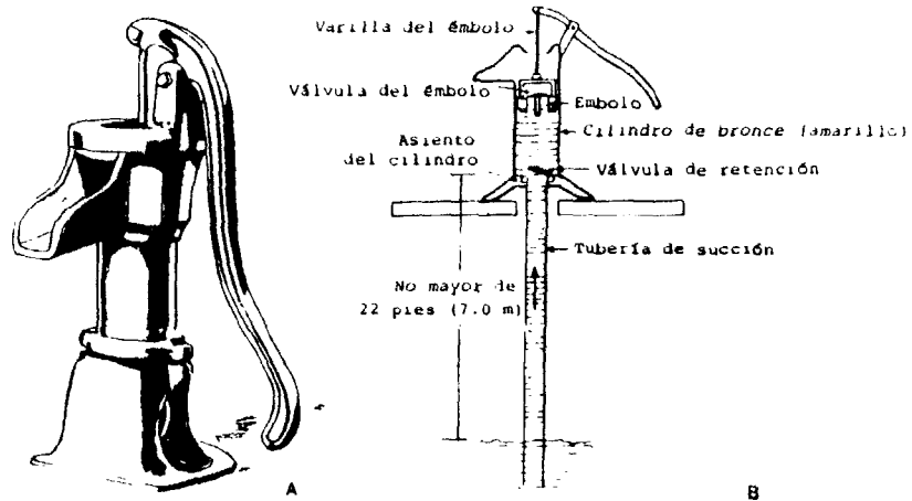
TIPICA BOMBA ASPIRANTE PARA POZO SUPERFICIAL
