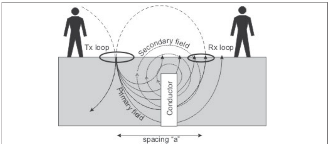
Figure 5.40: Slingram configuration (VD), EM 34.
